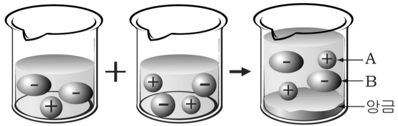
질산납 수용액 요오드화칼륨 수용액
