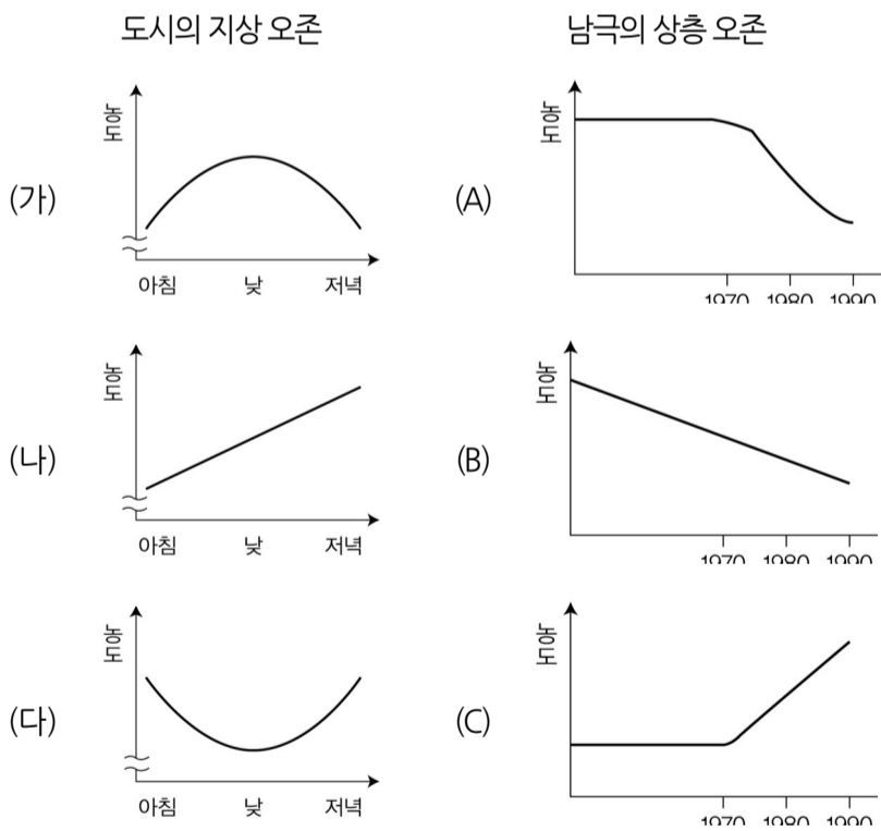
도시의 지상 오존 농도
